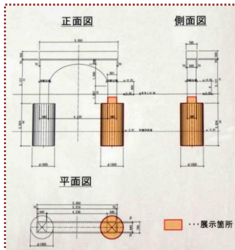
図-2 橋脚基礎の展示箇所
