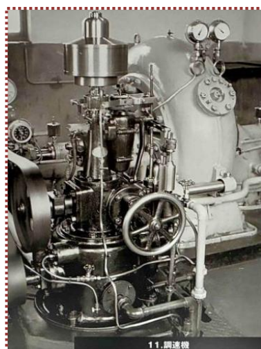
写真-10 调速機
