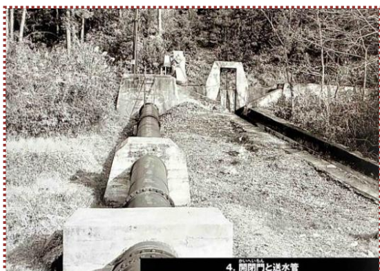
写真-6 開閉門と送水管
